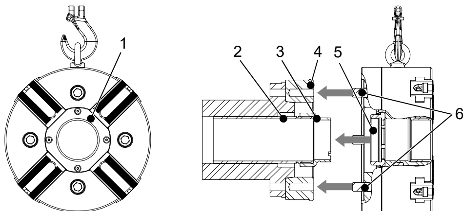
Fig. 3-4: Montaje del mandril de sujeción
